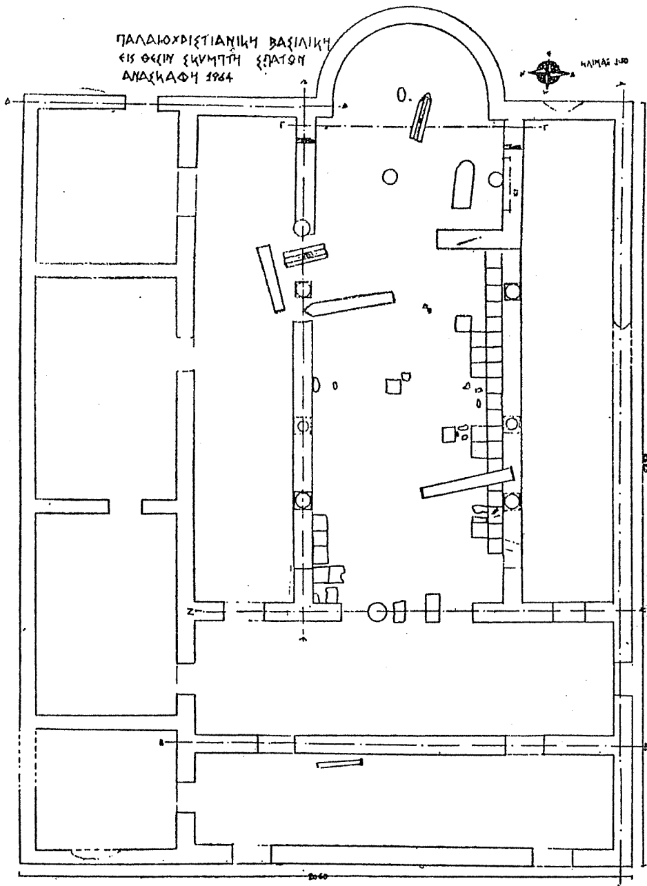
12. Βασιλική στη θέση Σκίμπι ή Σκίπθι των Σπάτων. Κάτοψη (Π. Λαζαρίδης)
