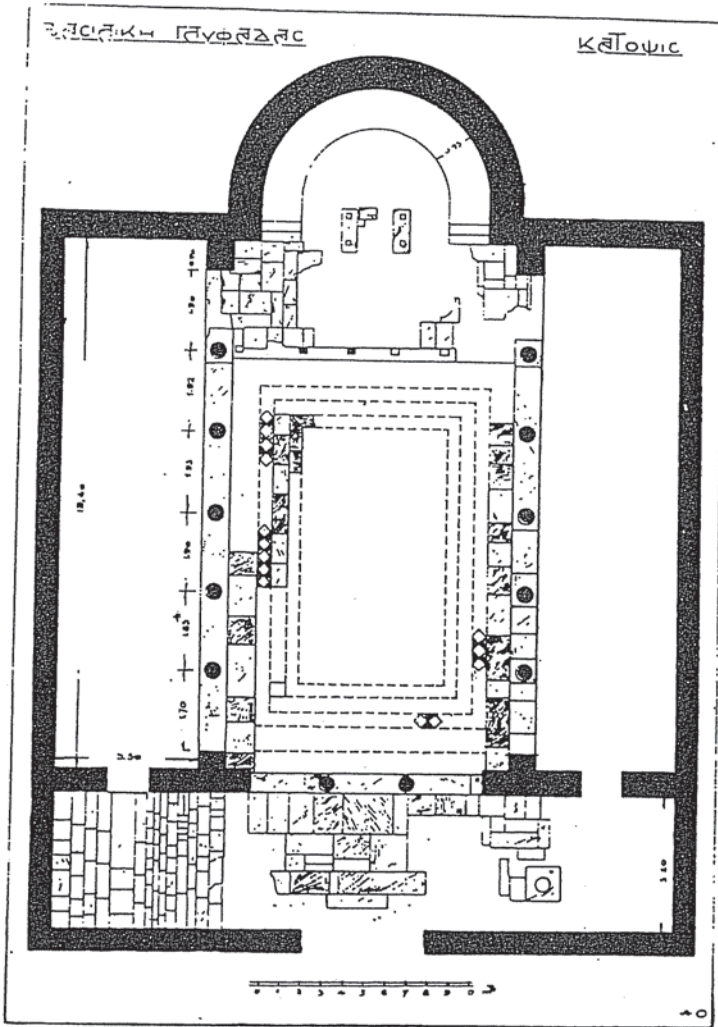
17. Βασιλική Γλυφάδας. Κάτοψη (Α.Κ. Ορλάνδος)
