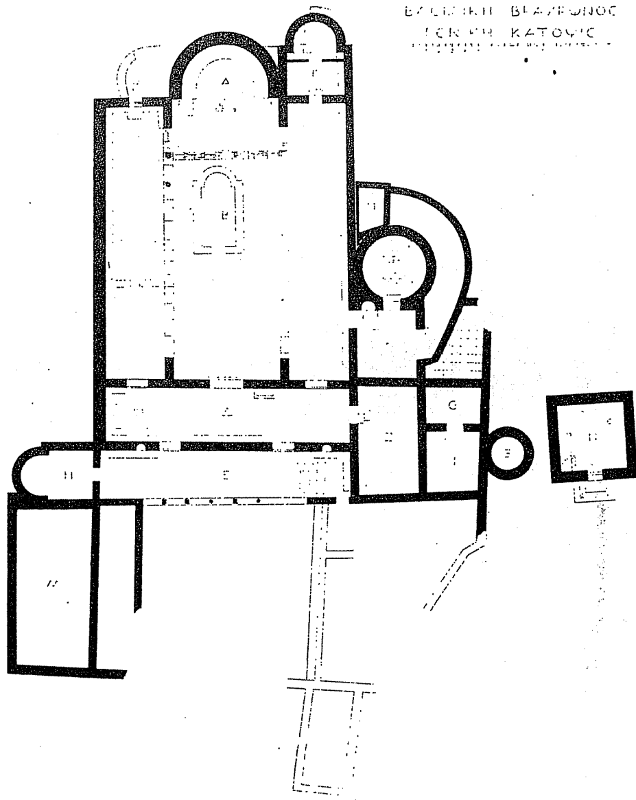
3. Βασιλική της ΒραΨώνας, Κάτοψη (Ε. Στίκας)
