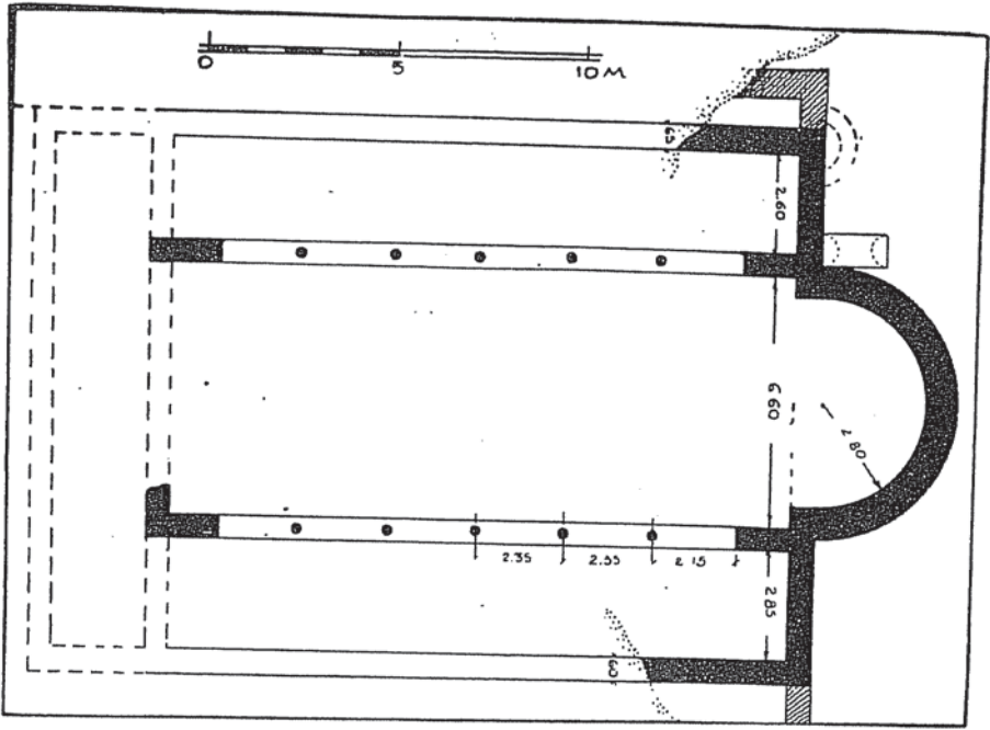
10. Βασιλική των Καλυβιών Κουβαρά. Κάτοψη (Α.Κ. Ορλάνδος)
